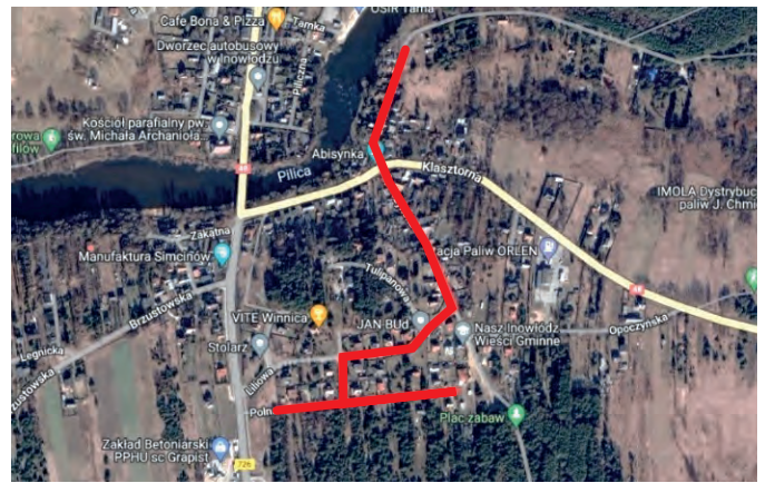
Budowa sieci kanalizacji w prawobrzeżnym Inowłodzu
