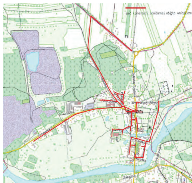
Sieć kanalizacji sanitarnej w Inowłodzu
